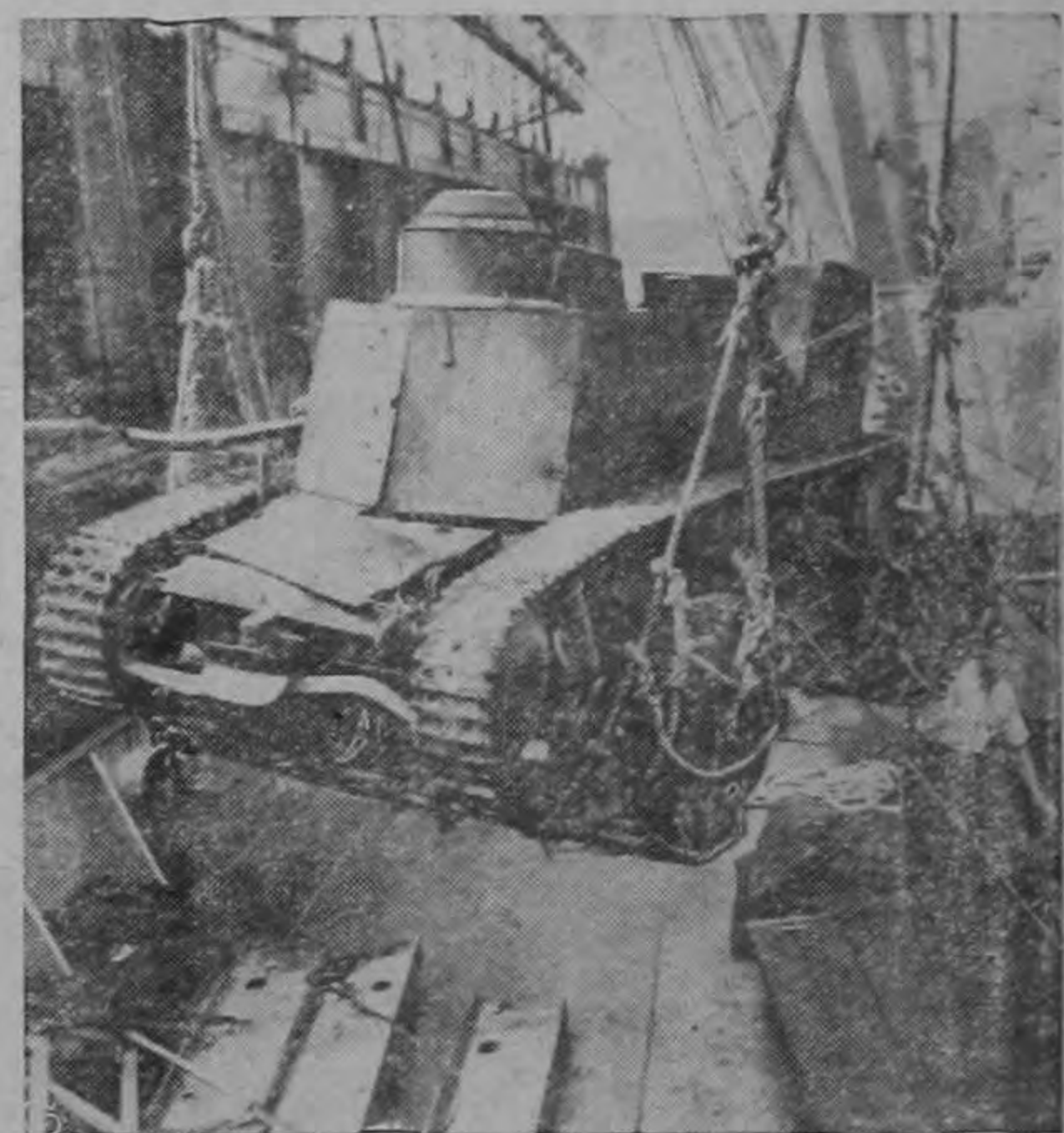
REPLICA AMERICANA del tanque de 5 toneladas que atravesó la Cortina de Hierro llevando 8 checoslovacos a la libertad el 25 de julio. Uno de los fugados, mecánico de Pilsen, trabajó durante 2 años secretamente, de noche, construyendo el vehículo con partes de automóvil y chatarra. El tanque que se desembarca en Nueva York, será exhibido en varios lugares de los Estados Unidos. (International).
